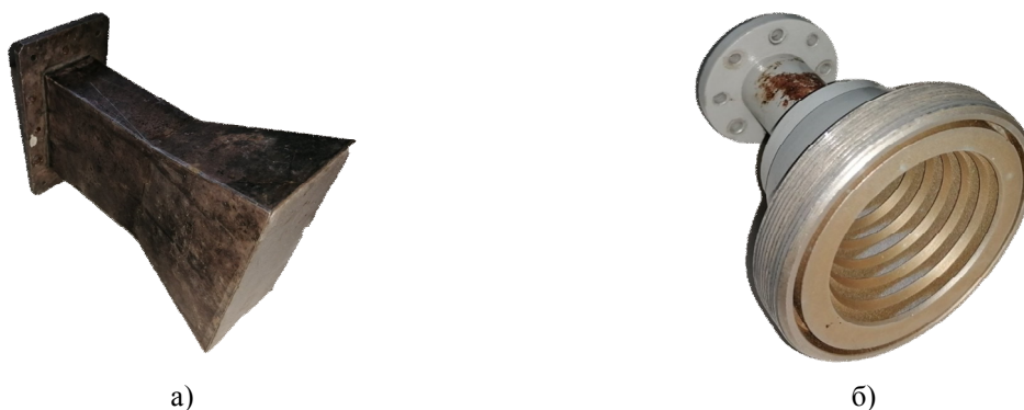
Рис. 3. Рупоры для генераторов шума: а) пирамидальный; б) конический гребенчатый
