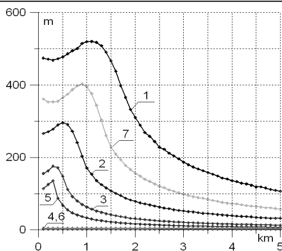
Рис. 6. SKO оценок высоты 7 разных целей при полосе сигнала 20 МГц
