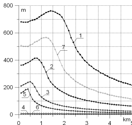
Рис. 4. SKO оценок высоты 7 разных целей при полосе сигнала 10 МГц
